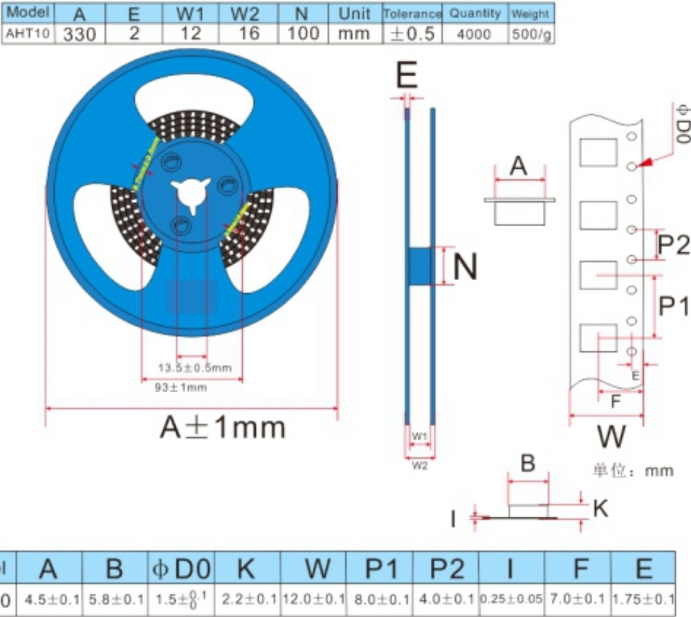
图20 包装卷带和传感器定位图
