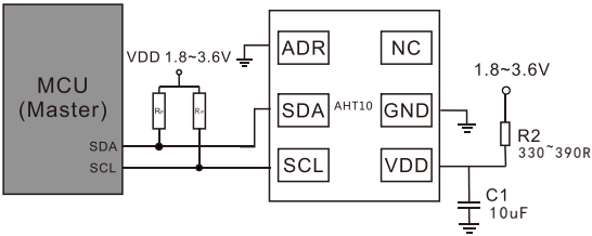
图 11 典型的应用电路，包括上拉电阻 RP 和 VDD 与 GND 之间的去耦电容。
