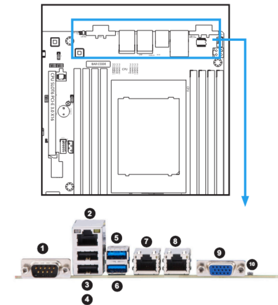
Рисунок 2-1. Расположение и определения портов ввода-вывода
