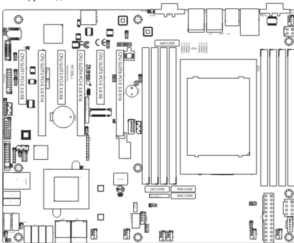
Рисунок 1-2. Компонировка серии материнских плат H11SSL
