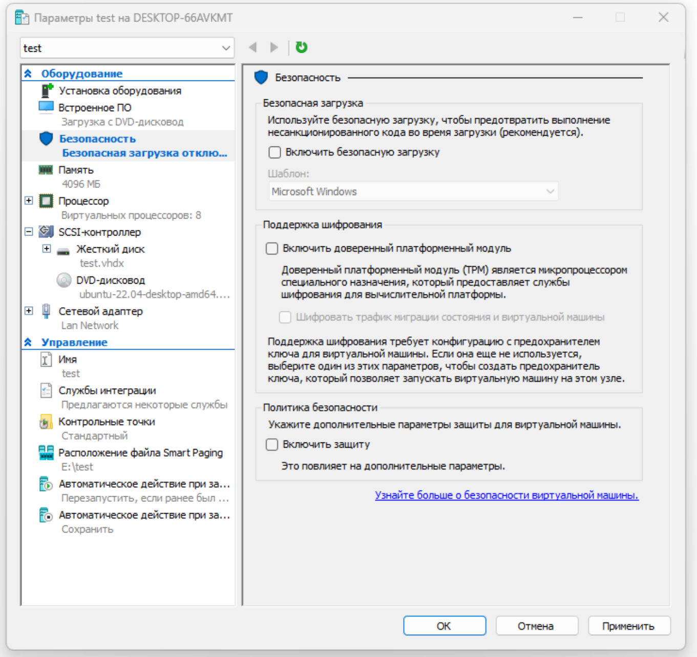
Во вкладке процессор указываем желаемое число виртуальных процессоров.
